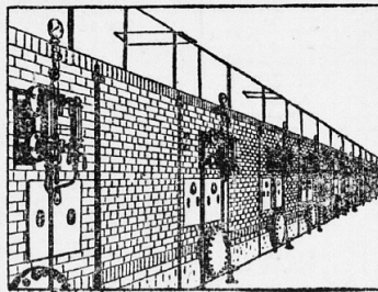
Einmauerung von 12 Zweiflammenrohrkesseln nach dem Bogensystem
