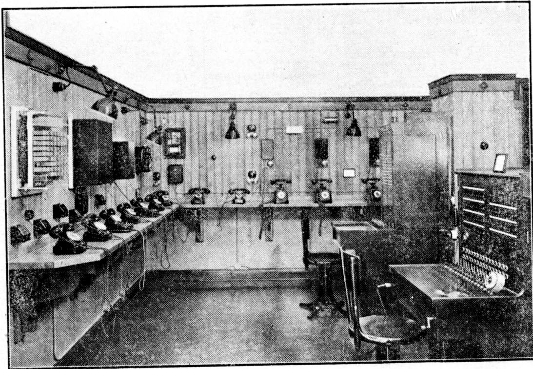
Ansicht aus dem Musterraum für Fernsprecheinrichtungen beim Fernsprechamt 2 Hamburg
