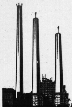
3 Schornsteine je 102.20 m hoch, 4.50 o. i. Durchm. für H.E.W. Kraftwerk Tiefstack
