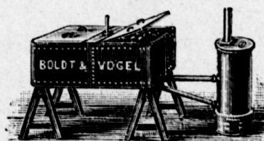
Pasteurisir-Apparat mit Heizofen. Fig. 219.
