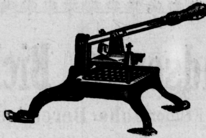
Kartoffelschneidemaschine.
