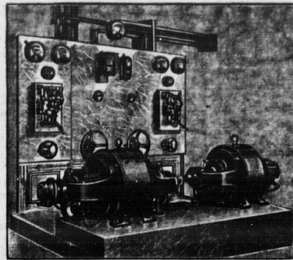
Einanker-Umformer-Anlage
