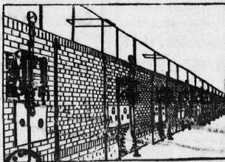
Einmauerung von 12 Zweiflammenrohrkesseln nach dem Bogensystem
