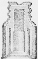
ISOLATOR im Querschnitt.
