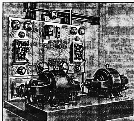
Einanker-Umformer-Anlage
