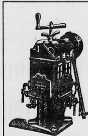
Vierstempelige Schmierpresse
