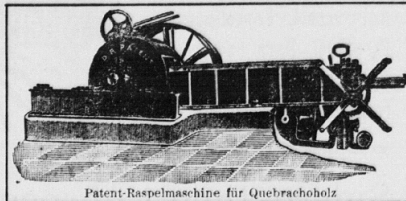
Patent-Raspelmaschine für Quebrachholz
