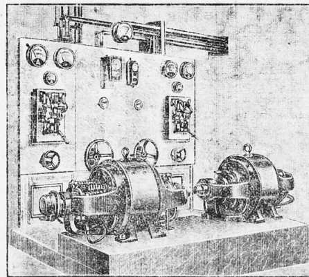
Einanker-Umformer-Anlage
