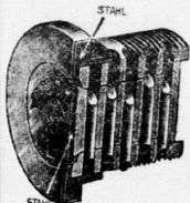
Schnitt durch den Croning-Zylinder
