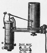
Der Crosby-Indikator.
