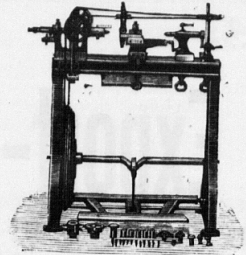
Patronendrehbank mit Rollenfräseinrichtung
