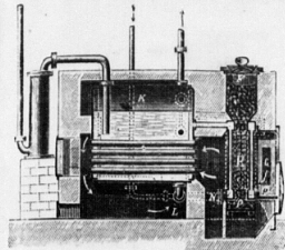
Körting'scher Niederdruck-Dampfkessel.
