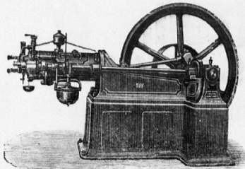
Otto's neuer Motor, liegd. Modell A.
