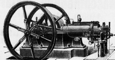
Körting'scher liegender Gasmotor.
